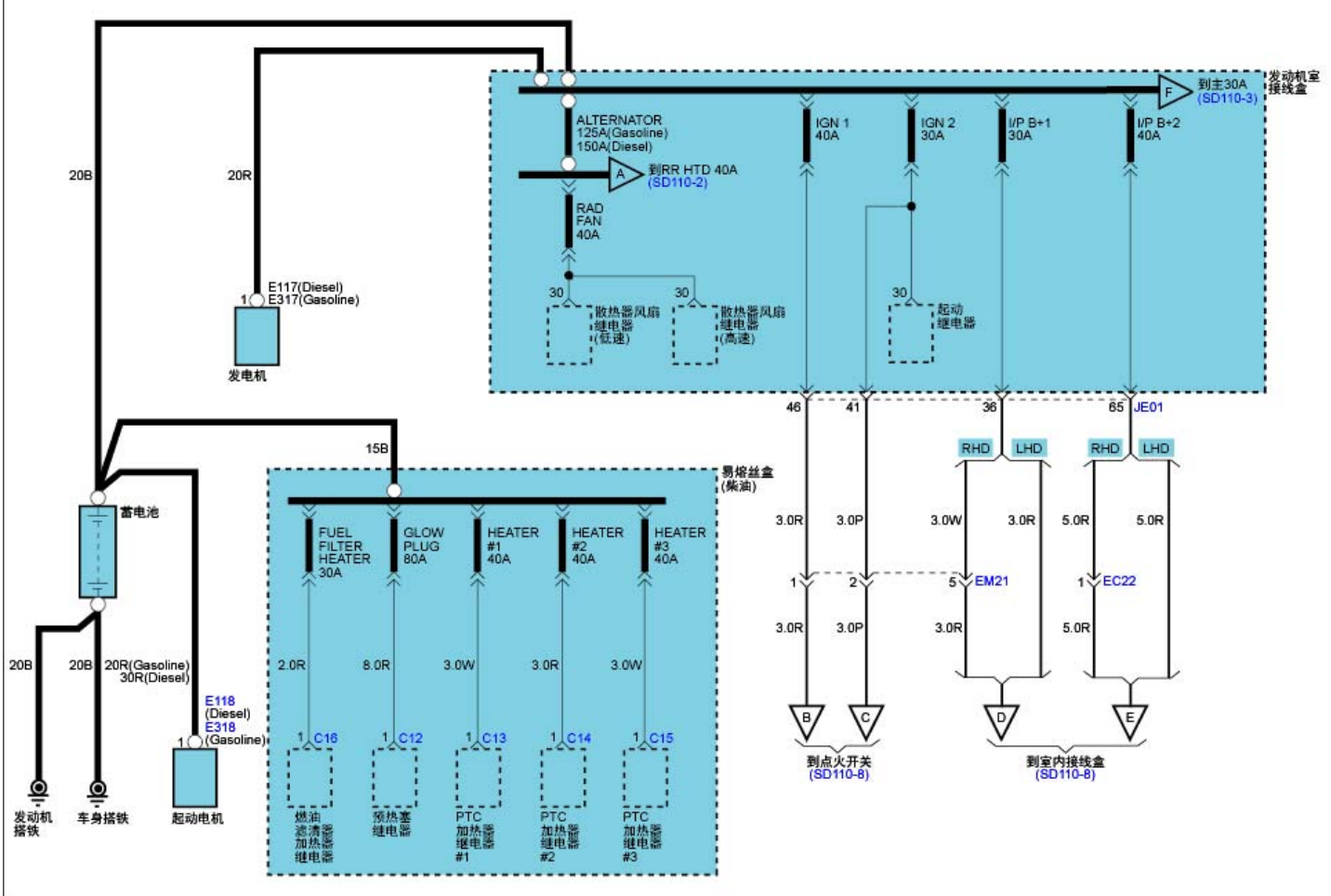
电源分布(1)
